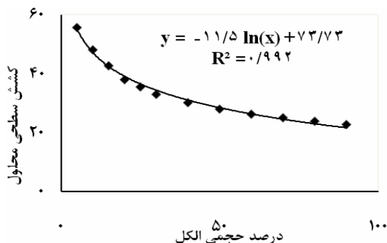
شکل ۲. رابطه بین درصد حجمی الکلی و کشش سطحی محلول آب-الکل (Vazquez et al., 1995)
